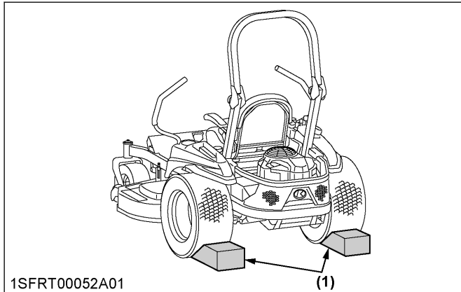
(1) Chock
